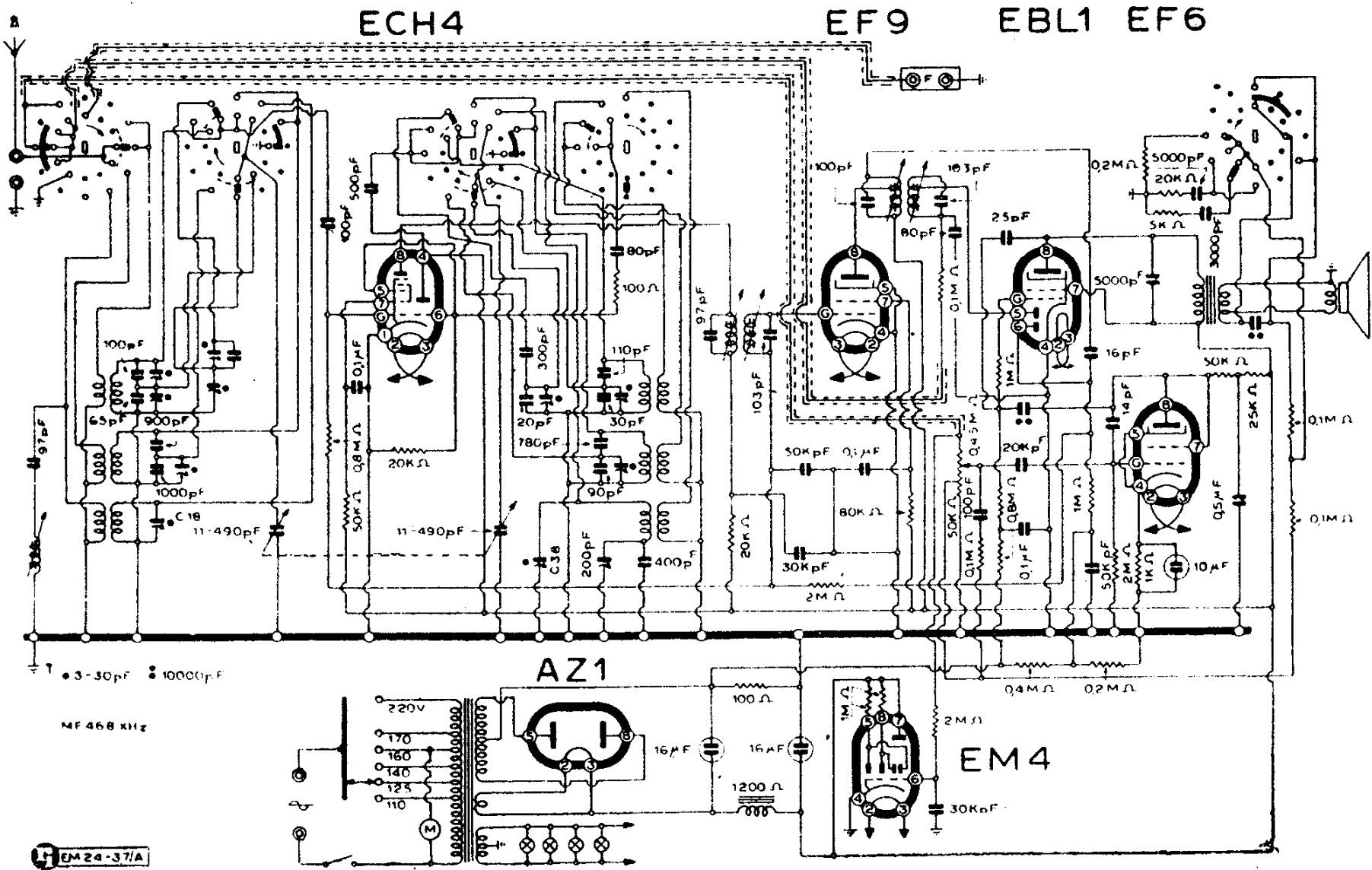
PHILIPS RADIO - MOD. « BI 580/A »
